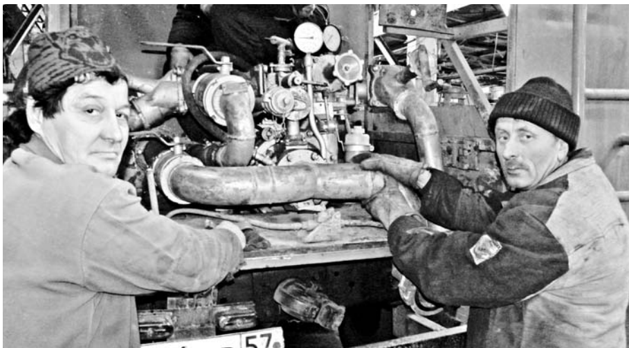
Механосборочный цех № 1 (цех по производству мотопомп МП-800Б). Слева направо: бригадир слесарей-монтажников Сергей Тимофеев, электросварщик Сергей Андреев.
